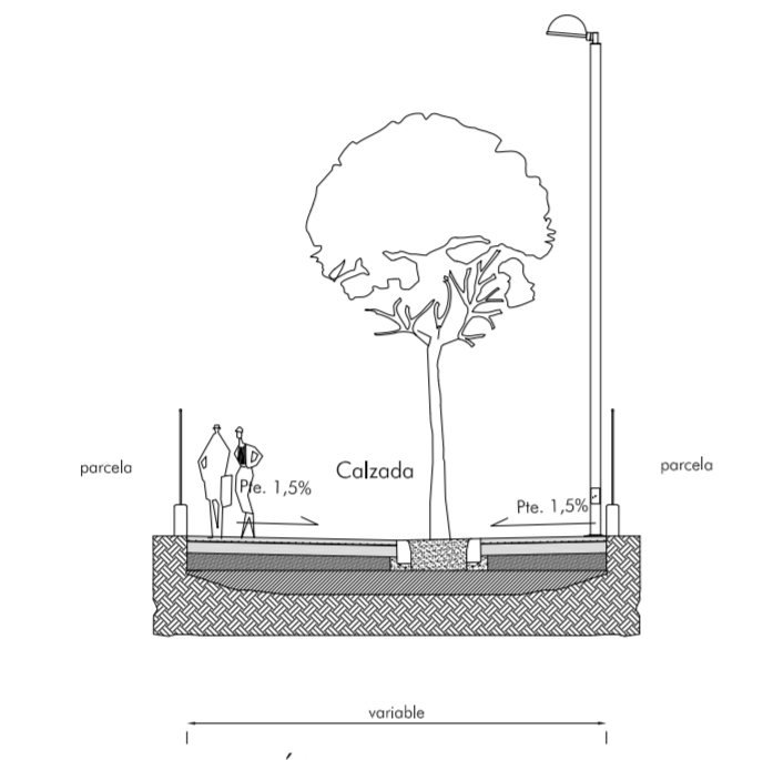
SECCIÓN 5
