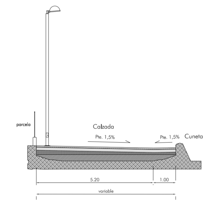
SECCIÓN 9
