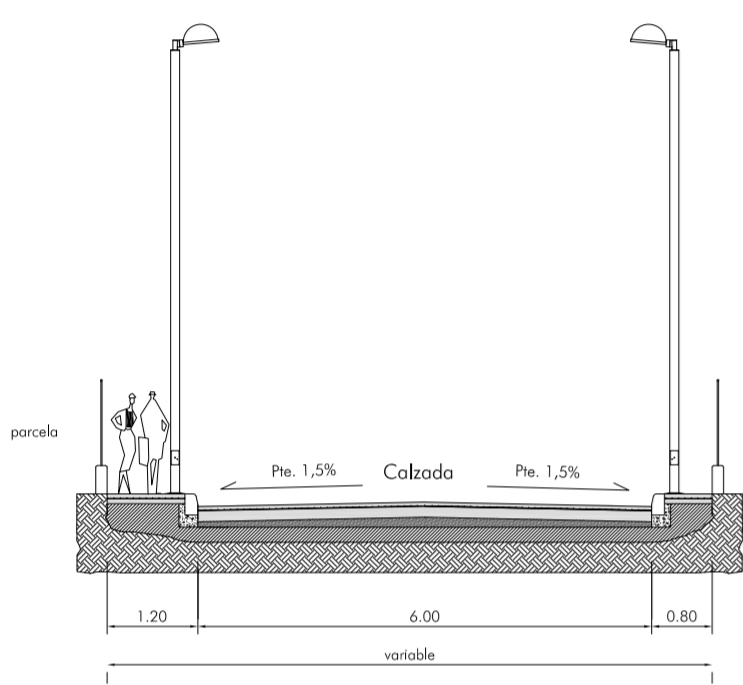
SECCIÓN 4
