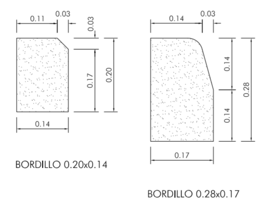
DETALLE BORDILLOS E 1_10
