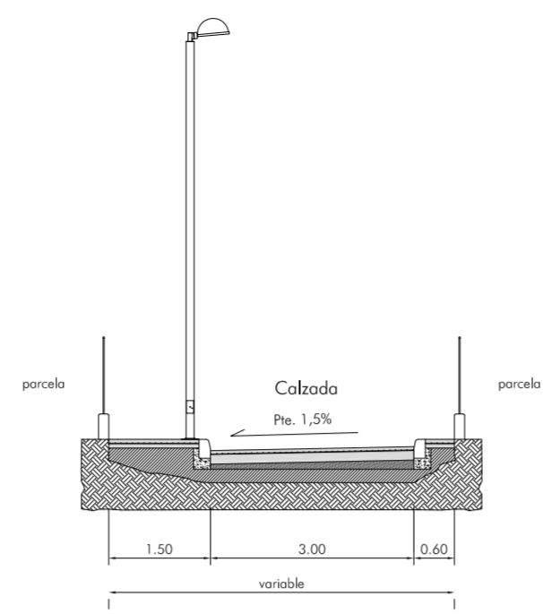
SECCIÓN 3
