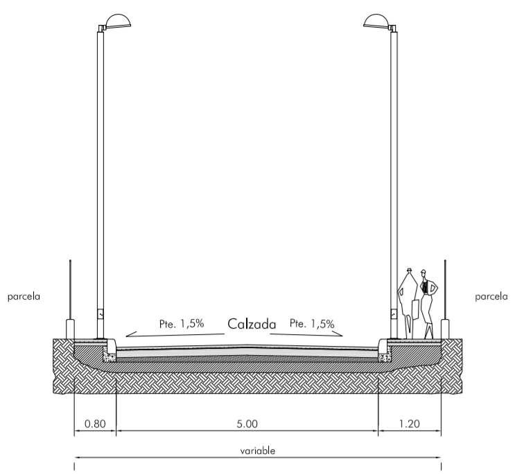
SECCIÓN 1
