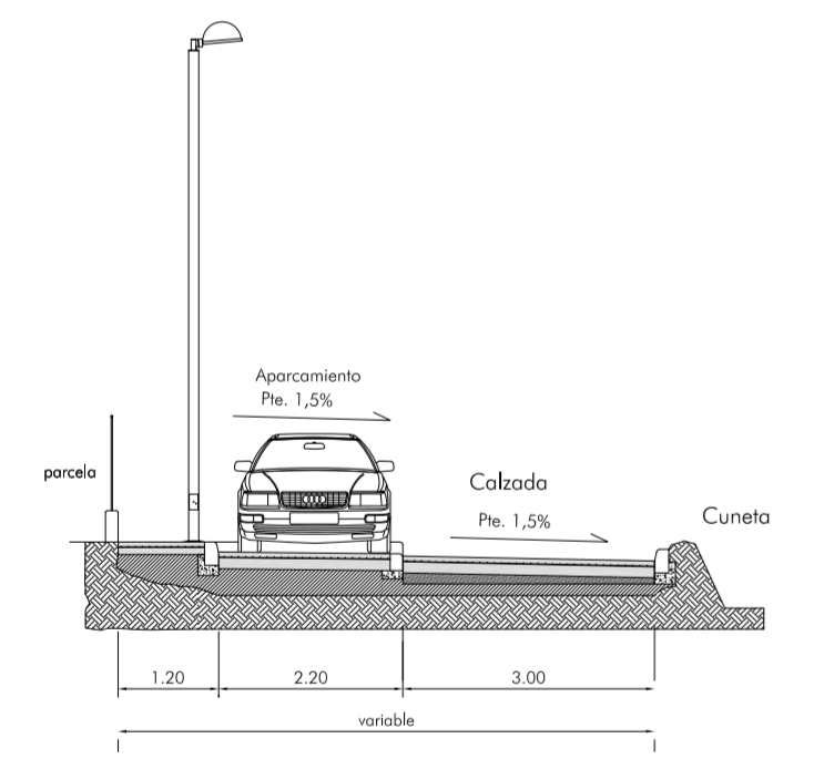
SECCIÓN 8
